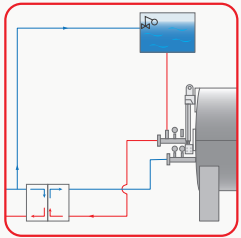
Geschlossener Wärmetauscher
